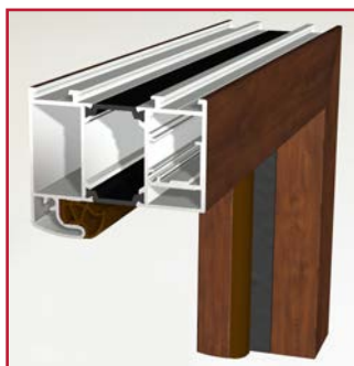
Hliníková zesílená zárubeň
