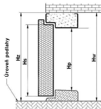
Vysvětlující vyobrazení zárubní a prahů: FAP SL, FRP SL, ALUTERM, FA SL s vložkou
