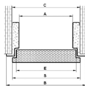
Vysvětlující vyobrazení zárubní a prahů: FTP SL
