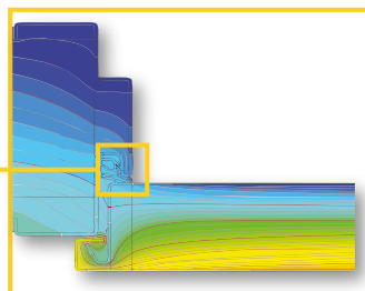
standardní zárubeň
