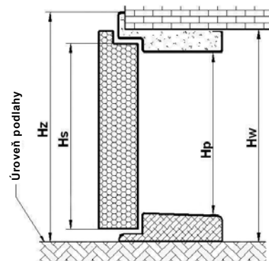
Vysvětlující vyobrazení zárubní a prahů: FTP SL
