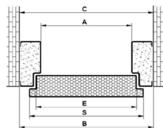
Vysvětlující vyobrazení zárubní a prahů: FAP SL, FRP SL, ALUTERM, FA SL s vložkou
